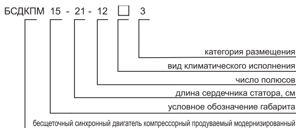
Структура условного обозначения двигателей типа БСДКПМ
