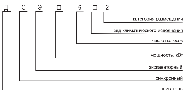
Структура условного обозначения двигателей серии ДСЭ-750, 630
