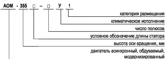
Структура условного обозначения двигателей типа АОМ
