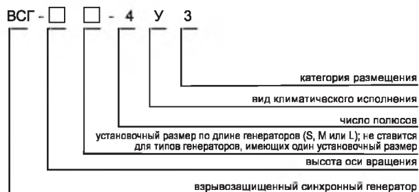
Структура условного обозначения генераторов синхронных типа ВСГ
