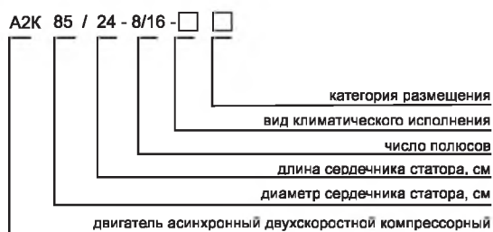
Структура условного обозначения двигателей типа А2К
